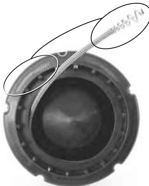
Kuva 20 - Kelaa jousi MYÖTÄPÄIVÄÄN, kun lataat jousen sisärummulle
