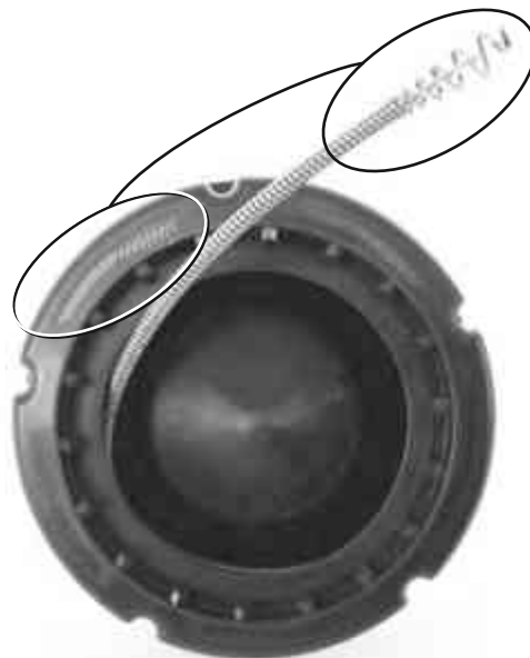
Slika 20 – Kad uvlačite sajlu u unutarnji bubanj, namotajte je U SMJERU KAZALJKE NA SATU
