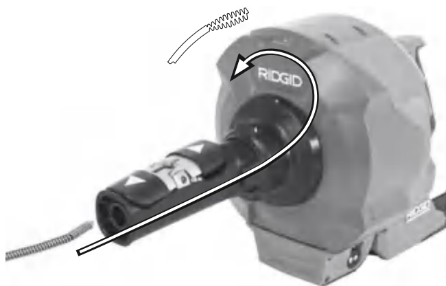
Afbeelding 21 – Veer laden zonder de binnentrommel te vervangen
