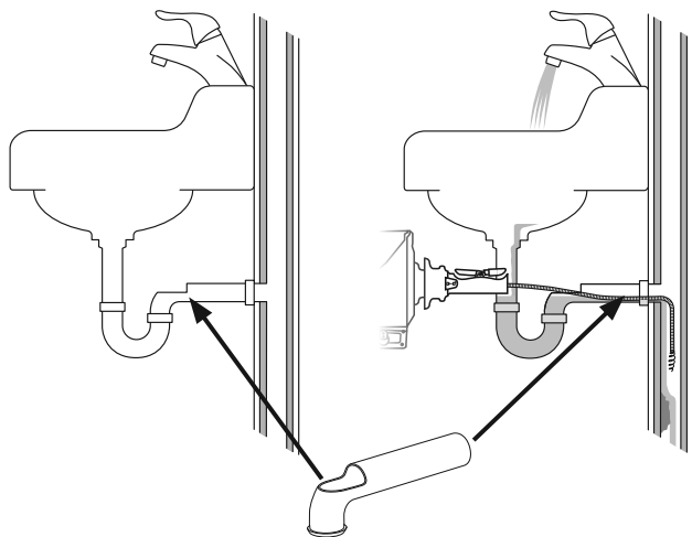
Figura 5 – Instalarea țevii de perete (accesoriu disponibil)
