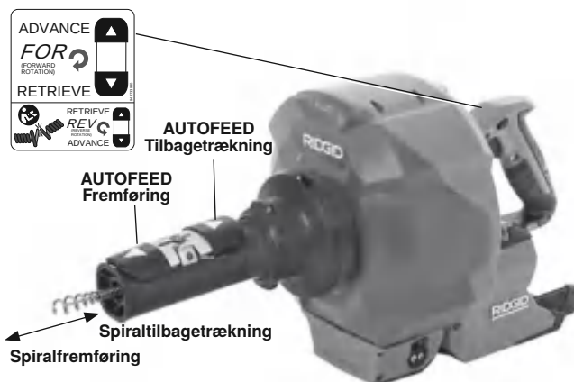
Figur 11 – AUTOFEED-enhedens betjeningslementer
