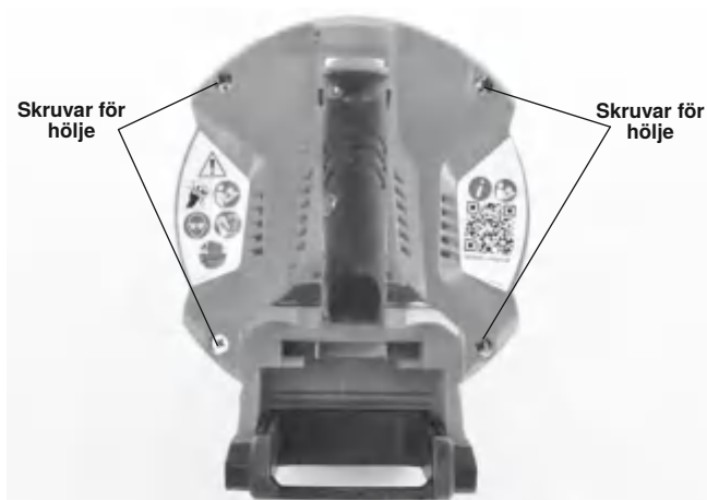
Figur 17 – Höljesskruvar
