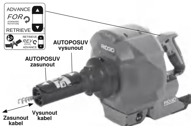
Obrázek 11 – Ovládací prvky jednotky AUTOPOSUVU
