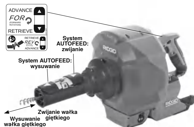
Rysunek 11 – elementy sterujące systemu AUTOFEED
