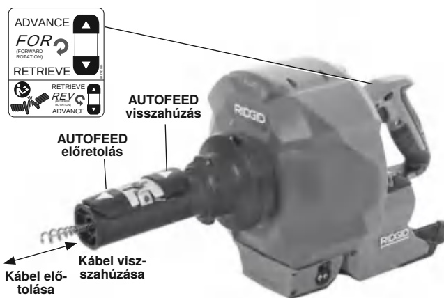
11. ábra - AUTOFEED egység kezelőszervei
