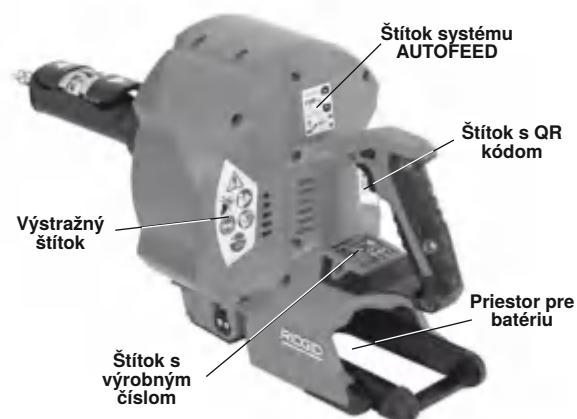
Obrázok 1B – Drezová batérová čistička RIDGID® K-46
