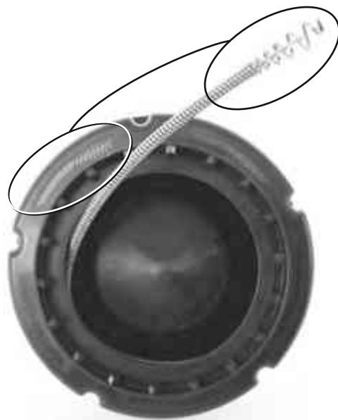
Figura 20 - Caricare il cavo in un tamburo interno avvolgendolo in senso ORARIO
