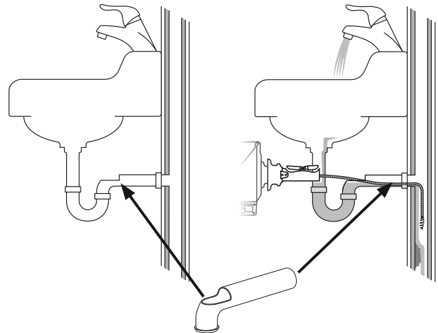
Afbeelding 5 – Installatie wandbuis (verkrijgbaar als accessoire)
