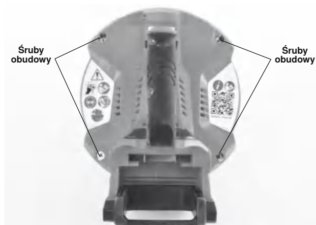
Rysunek 17 – śruby obudowy
