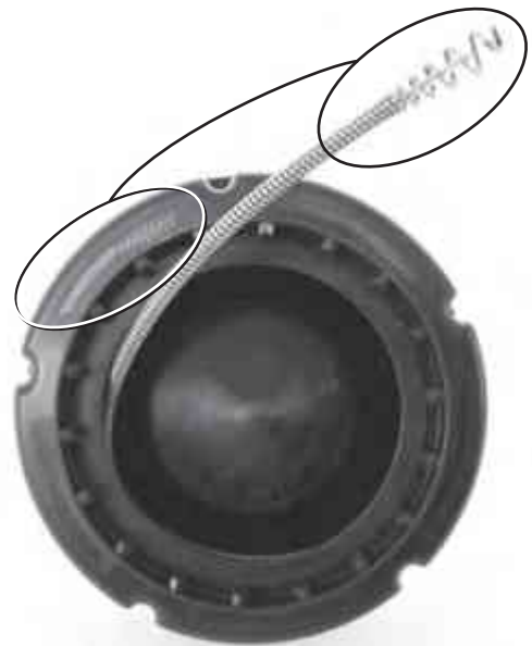
図 20 - ケーブルを内部ドラムに収納する際は、ケーブルを時計回りに巻き入れる
