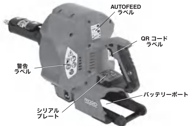
図 1B – RIDGID® K-46 Cordless SinkSnake
