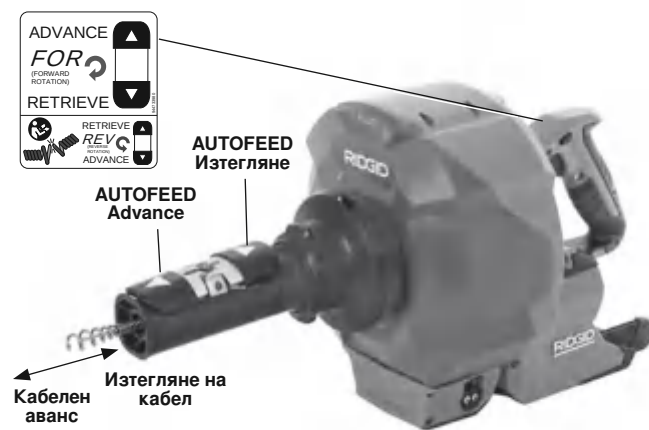
Фигура 11 - Управление на AUTOFEED блока
