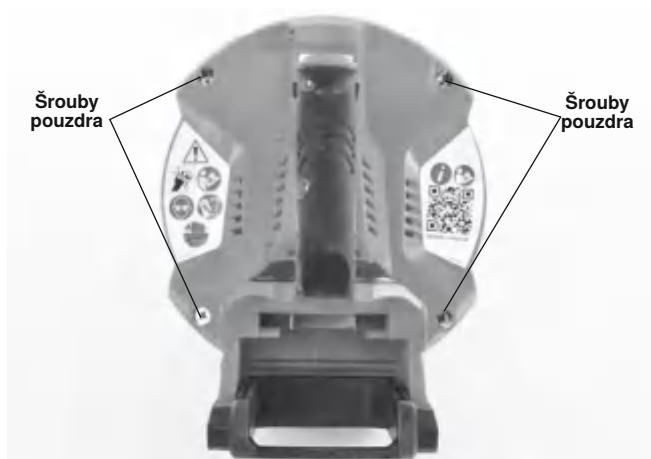
Obrázek 17 – Šrouby krytu
