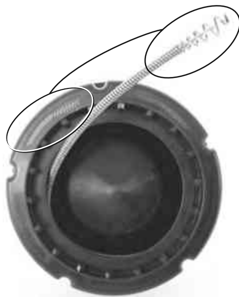
Figura 20 – Când încărcați cablul pe un tambur interior, înfășurați cablul ÎN SENS ORAR
