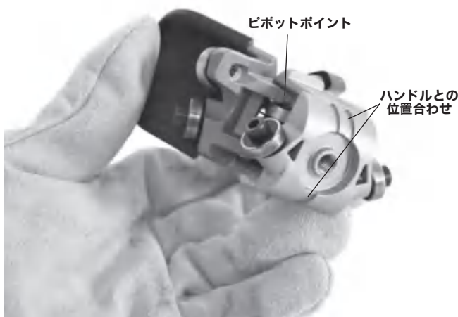
図 16B – AUTOFEED 機構
