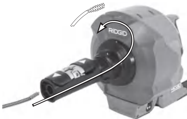
Abbildung 21 – Einlegen der Spirale ohne Wechsel der Innentrommel
