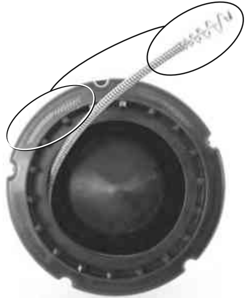
Εικόνα 20 – Κατά την τοποθέτηση του σπιράλ μέσα στο εσωτερικό τύμπανο, τυλίξτε το σπιράλ ΔΕΞΙΟΣΤΡΟΦΑ
