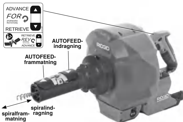
Figur 11 – AUTOFEED-enhetens reglage
