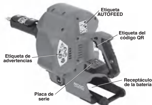
Figura 1 B – Limpiaadora K-46 SinkSnake sin cordón de RIDGID®
