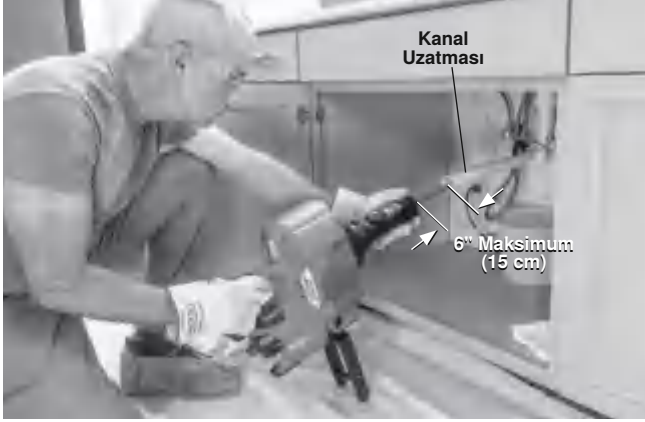
Şekil 6 – Drenajın AUTOFEED Ünitesinin 6" (15 cm) İçine Kadar Uzatılmasına Örnek
