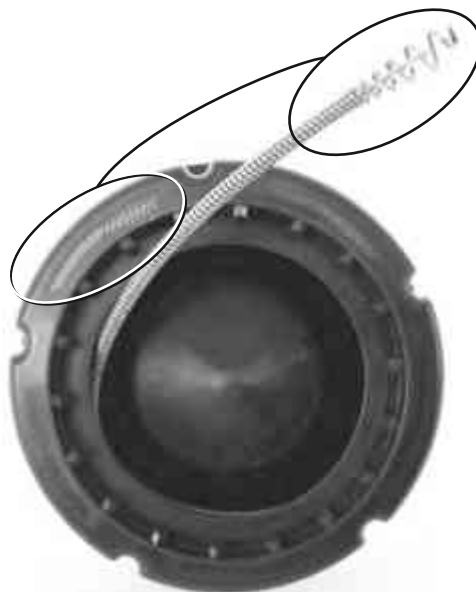
Figura 20 – Ao carregar o cabo para dentro do tambor interior, enrole-o rodando PARA A DIREITA
