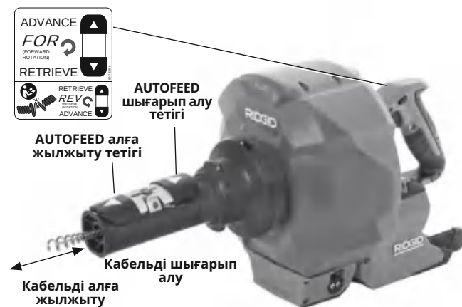
11-сурет – AUTOFEED бөлігінің басқару тетіктері
