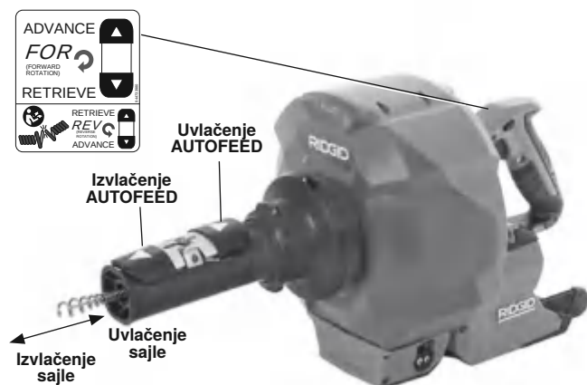
Slika 11 – Kontrole jedinice AUTOFEED
