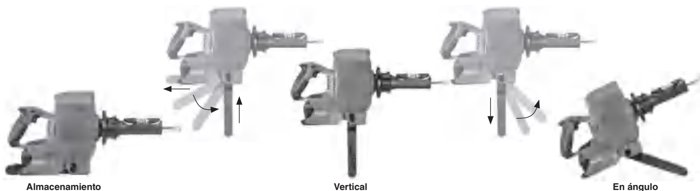
Figura 8 – Ajuste de la base de soporte
