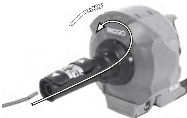
Obrázek 21 – Navíjení kabelu bez výměny vnitřního bubnu
