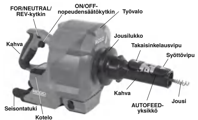
Kuva 1A - Johdoton RIDGID® K-46 Cordless SinkSnake -viemärinavaaja
