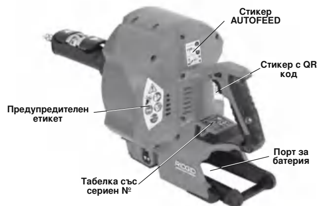
Фигура 1B – RIDGID® K-46 Cordless SinkSnake
