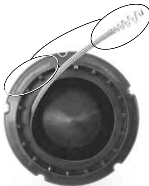
Рисунок 20 – При заправке спирали во внутренний барабан наматывайте спираль ПО ЧАСОВОЙ СТРЕЛКЕ
