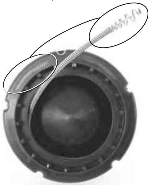
20-сурет – Кабельді ішкі барабанға салған кезде кабельді САҒАТ ТІЛІНІҢ БАҒЫТЫМЕН орау
