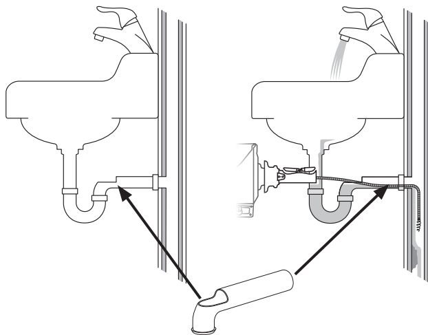
图 5 - 壁管安装（可用附件）
