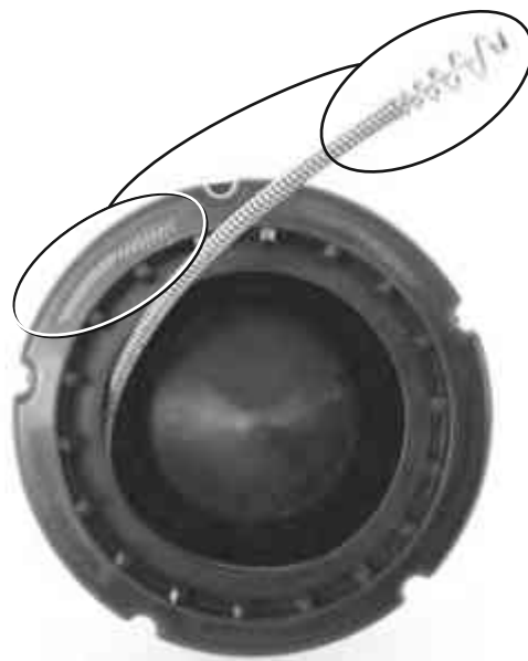
Obrázok 20 – Pri zavádzaní kábla do vnútorného bubna kábel navíjajte V SMERE HODINOVÝCH RUČÍČIEK
