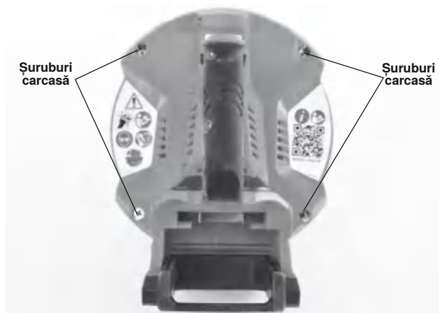
Figura 17 – Șuruburile carcasei
