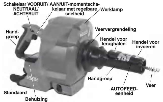
Afbeelding 1A – RIDGID® K-46 Draadloze SinkSnake
