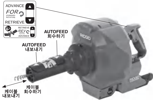
그림 11 - AUTOFEED 장치 제어
