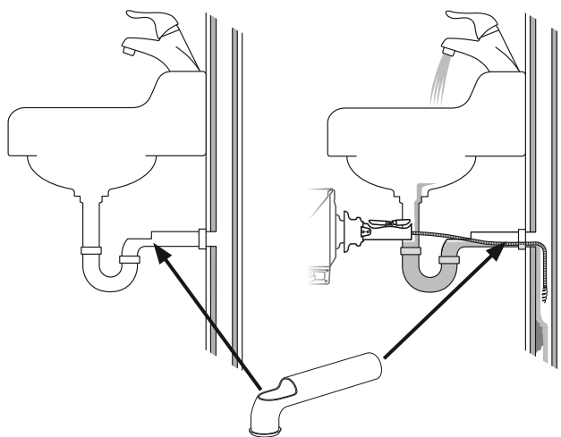
Slika 5 – Montaža zidne cevi (dostupni dodatak)
