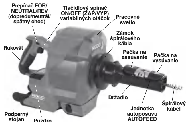
Obrázok 1A – Drezová batérová čistička RIDGID® K-46
