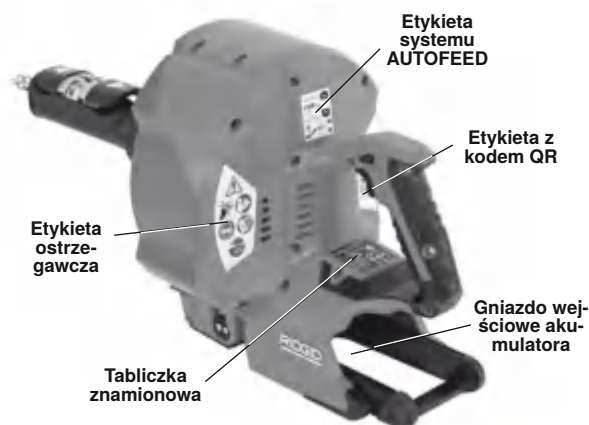
Rysunek 1B – bezprzewodowe urządzenie do czyszczenia odpływów RIDGID® SinkSnake K-46
