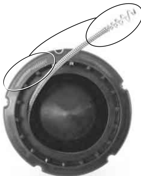
Rysunek 20 – Ładując wałek giętki do wewnętrznego bębna, zwinąć go W KIERUNKU ZGODNYM Z RUCHEM WSKAZÓWEK ZEGARA.
