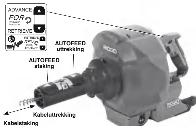
Figur 11 – AUTOFEED-enhetens kontroller
