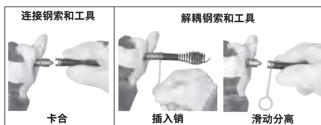
图 7 – 接头和解耦工具
