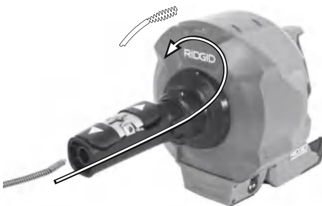
Figura 21 - Caricamento del cavo senza sostituire il tamburo interno
