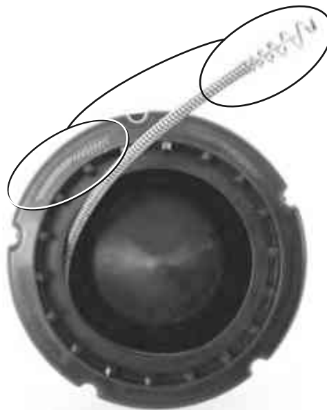
Figur 20 – När du lägger på spiral på en innertrumma ska spiralen lindas MEDURS
