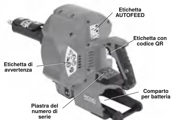
Figura 1B - Stasatrice per lavandini cordless K-46 RIDGID®
