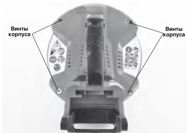
Рисунок 17 – Винты крепления корпуса
