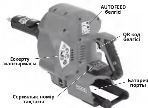
1B суреті – RIDGID® K-46 Cordless SinkSnake
