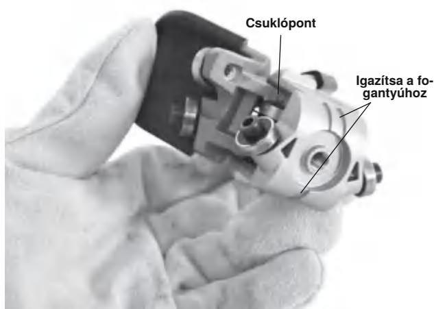
16B ábra - AUTOFEED mechanizmus
