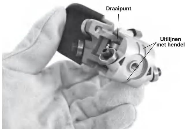
Afbeelding 16B – AUTOFEED-mechanisme
