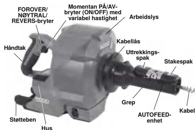
Figur 1A – RIDGID® K-46 Trådløs SinkSnake
