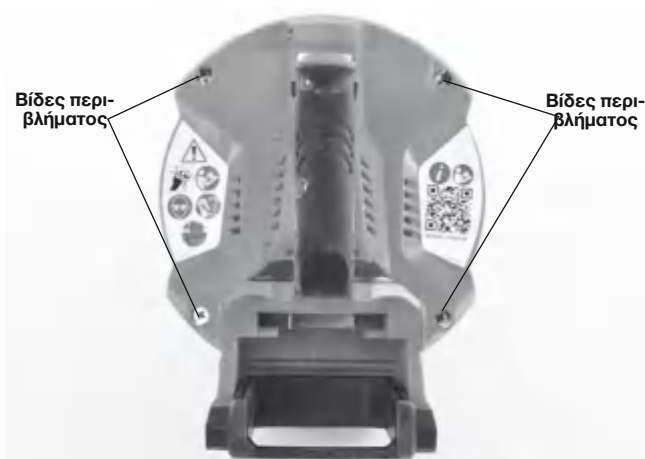
Εικόνα 17 - Βίδες περιβλήματος
