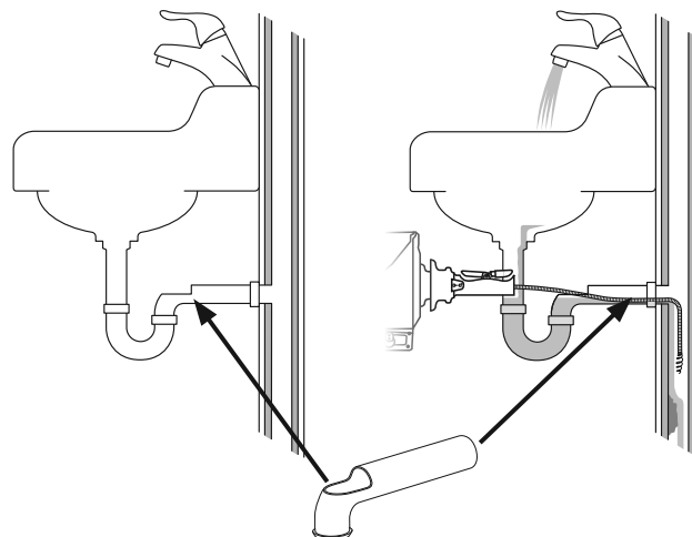
Rysunek 5 – Instalacja rury ściennnej (dostępne akcesoria)
