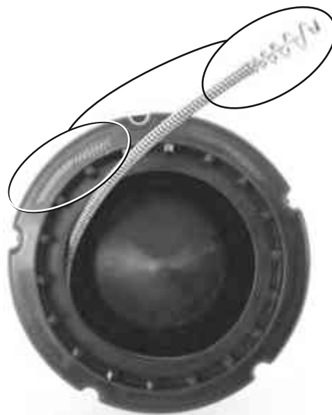
20. ábra - A belső dobba való kábeltekercselésnél az ÓRAMUTATÓ IRÁNYÁBA tekerjelen.
