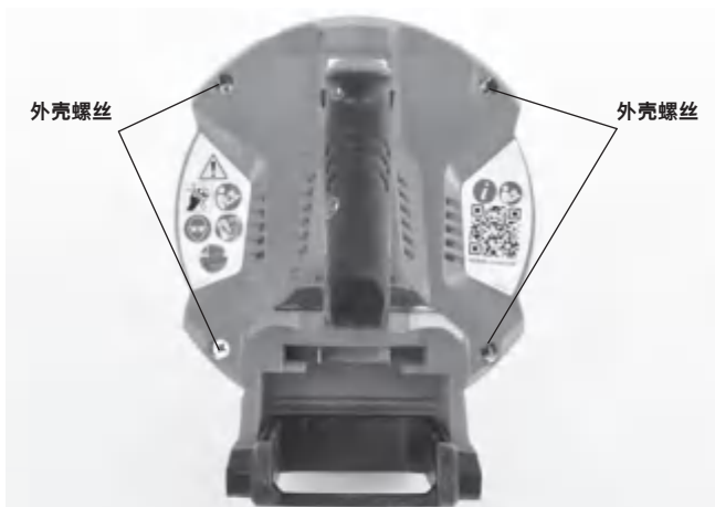
图 17 - 外壳螺丝
