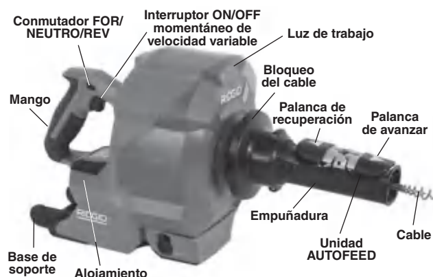
Figura 1 A – Limpiaadora K-46 SinkSnake sin cordón de RIDGID®
