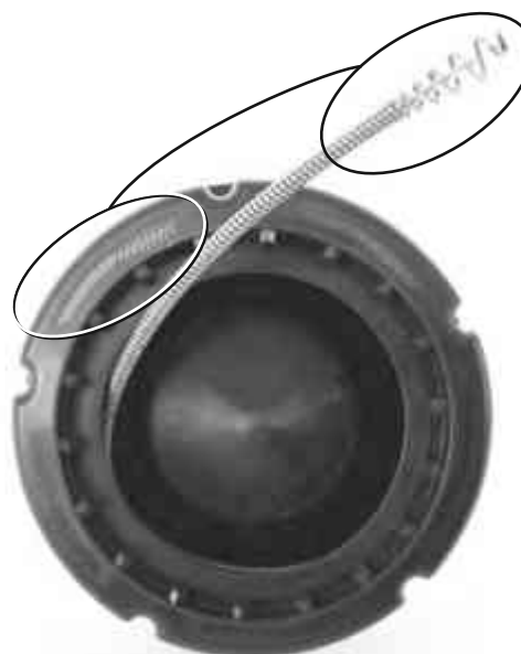
Obrázek 20 – Při navíjení kabelu do vnitřního bubnu kabel navíjejte VE SMĚRU HODINOVÝCH RUČÍČEK
