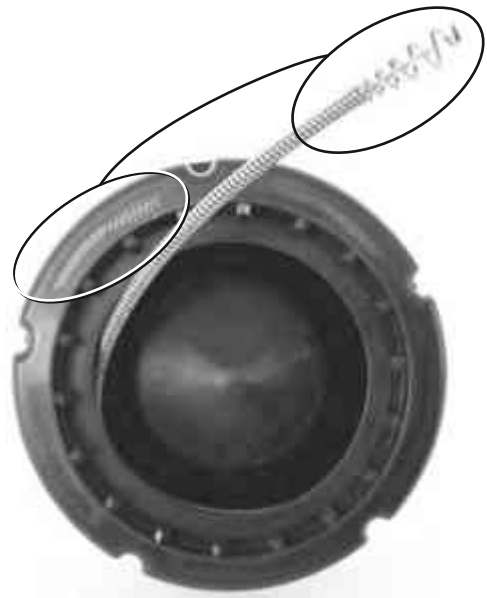
Afbeelding 20 – Wanneer u de veer in de binnentrommel aanbrengt, moet u de veer RECHTSOM in de trommel opwickelen
