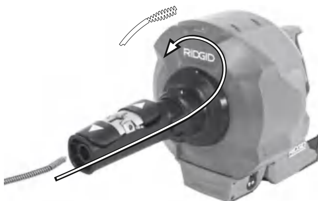
Rysunek 21 – Ładowanie sprężyny bez wymiany wewnętrznego bębna
