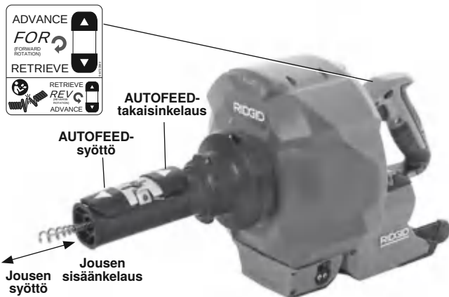
Kuva 11 - AUTOFEED-yksikön säätimet
