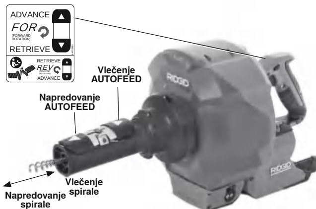
Slika 11 – Krmilniki enote AUTOFEED
