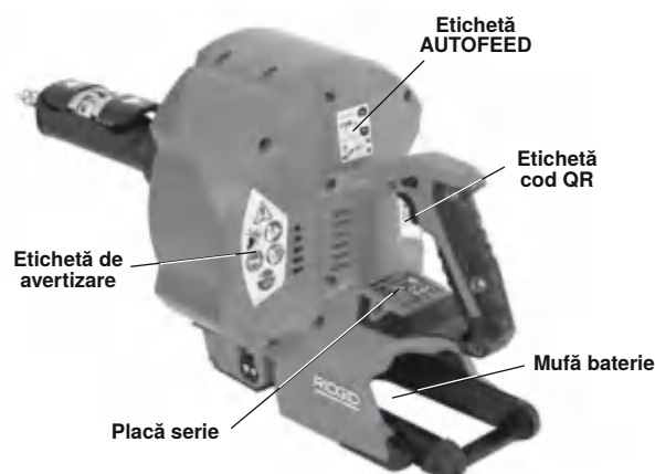
Figura 1B – RIDGID® K-46 SinkSnake fără fir
