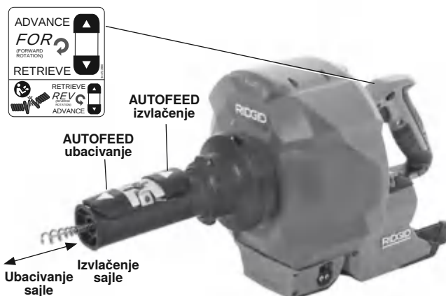
Slika 11 – Komande AUTOFEED jedinice
