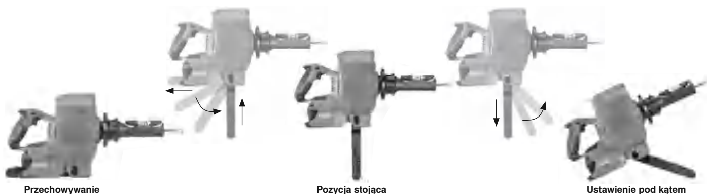
Rysunek 8 – regulowanie statywu
