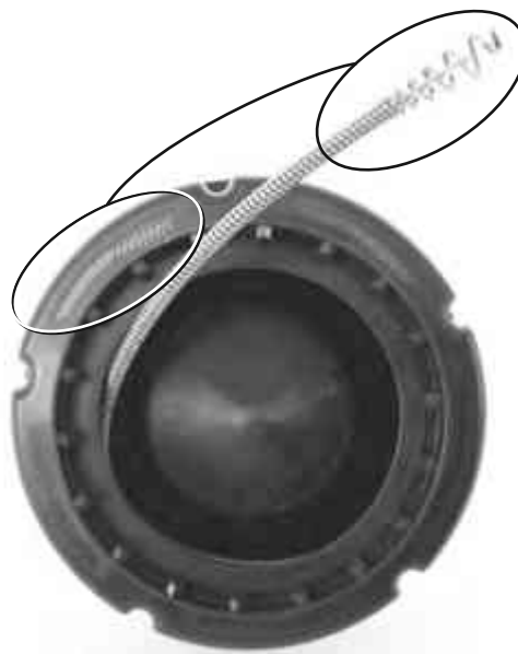
Slika 20 – Kada uvlačite sajlu u unutrašnji bubanj, namotavajte sajlu UDESNO
