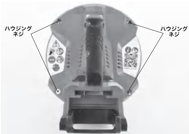
図 17 - ハウジングネジ
