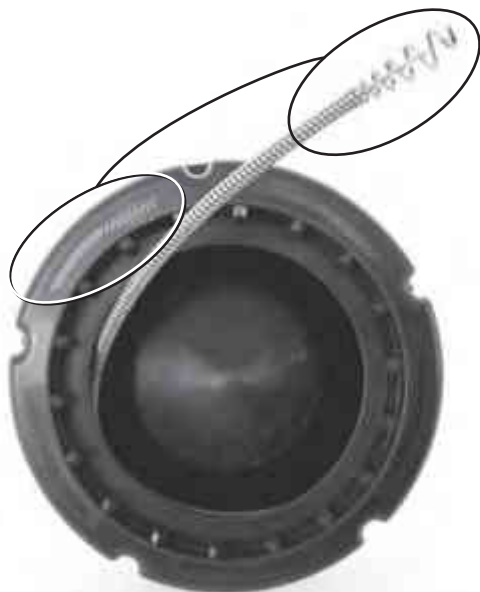
Abbildung 20 – Beim Einlegen der Spirale in eine Innentrommel die Spirale im Uhrzeigersinn aufwickeln
