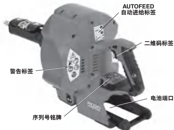
图 1B — RIDGID® 里奇 K-46 无线 SinkSnake
