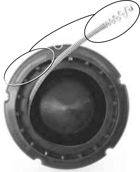
Şekil 20 – Kabloyu Bir İç Tambura Yüklerken, Kabloyu SAAT YÖNÜNDE Sarın
